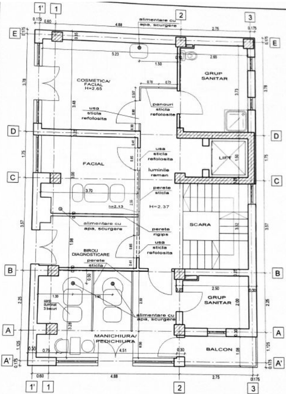
PLAN ETAJ 1 - PROPUNERE SC 1:50 Suprafata construita = 110,25 mp
