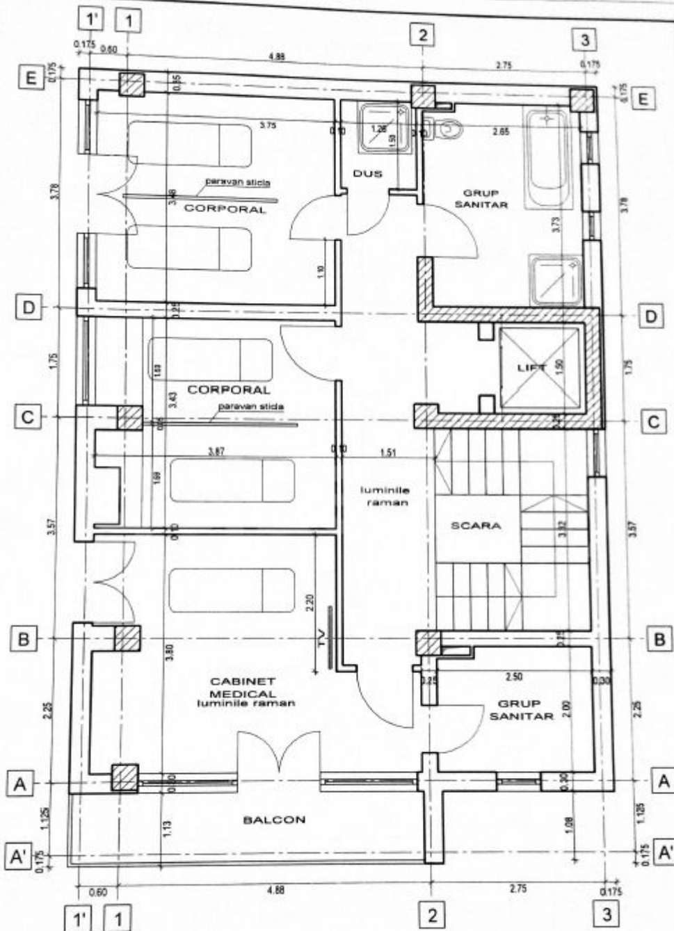
PLAN ETAJ 2 - PROPUNERE SC 1:50 Suprafata construita = 109,30 mp
