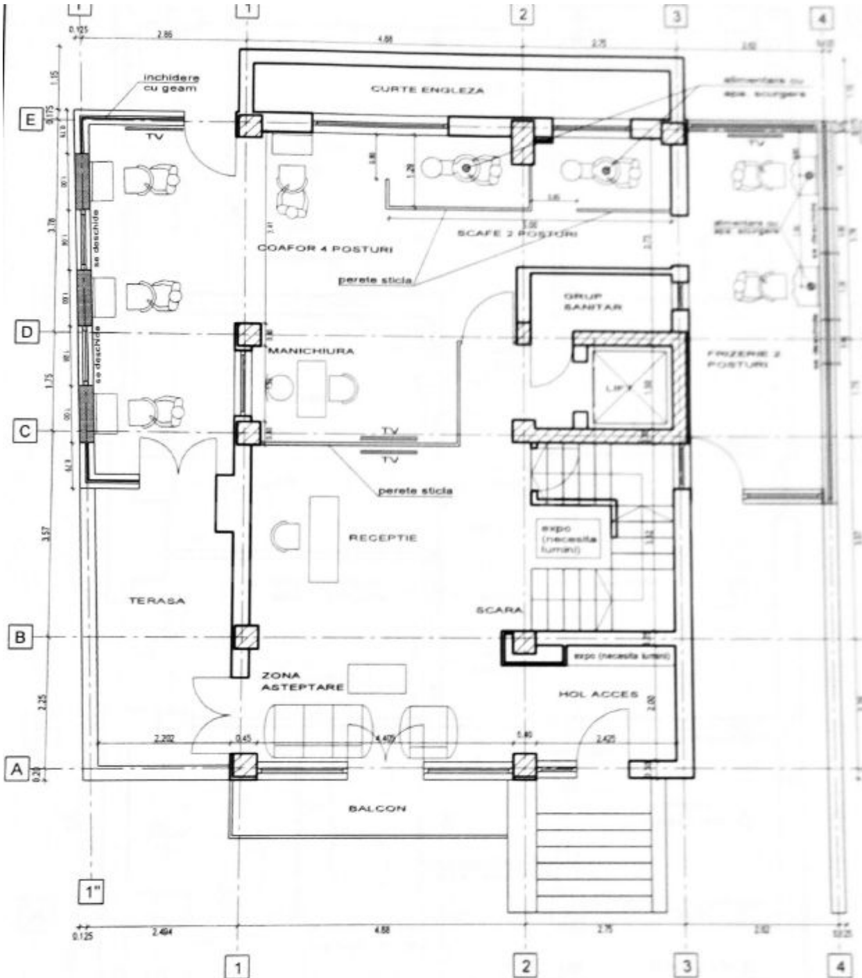
PLAN PARTER - PROPUNERE SC 1:50 Suprafata construita = 170,00 mp
