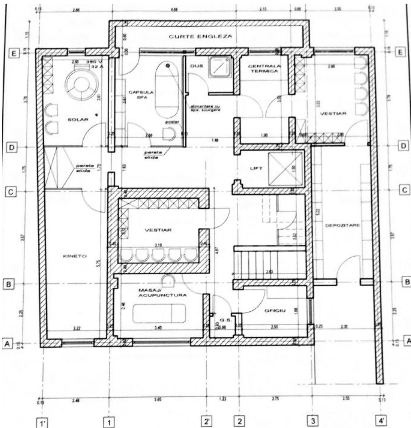
PLAN SUBSOL - PROPUNERE SC 1:50 Suprafata construita = 173 mp
