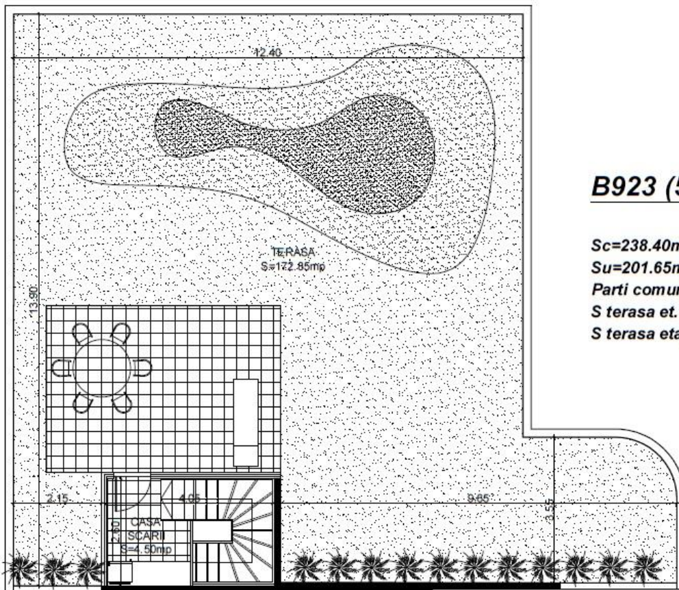
terasa
