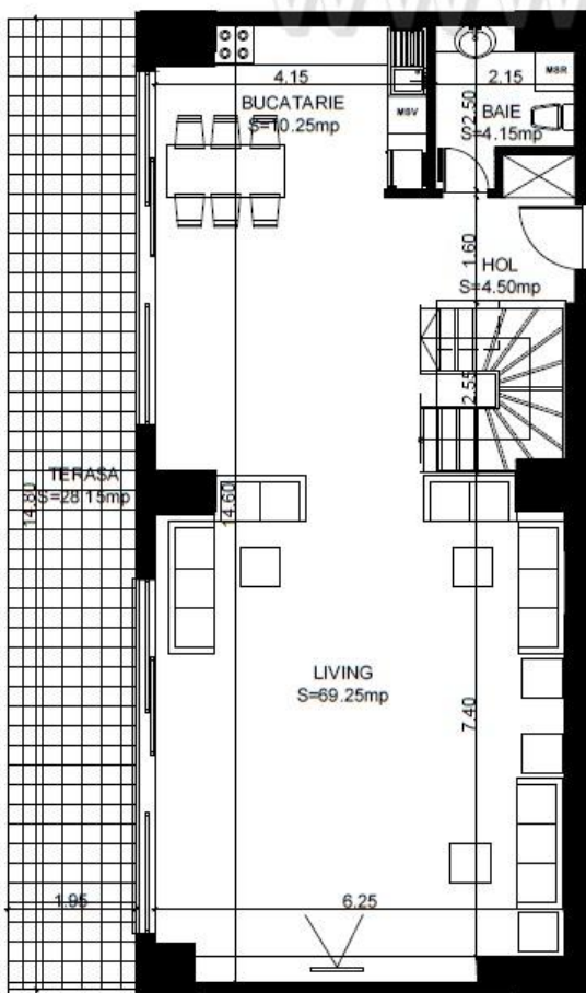
etaj 9
