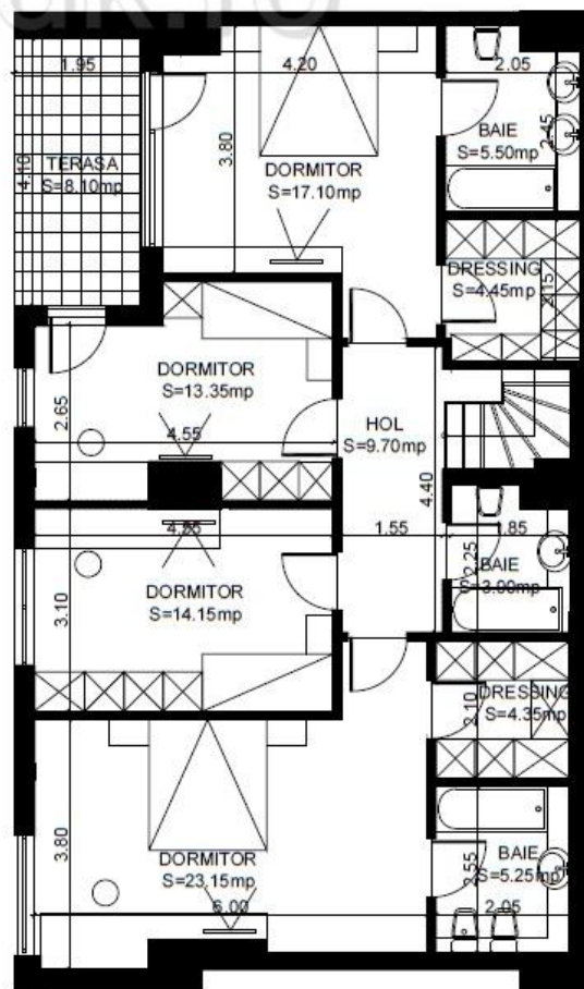
etaj 8
